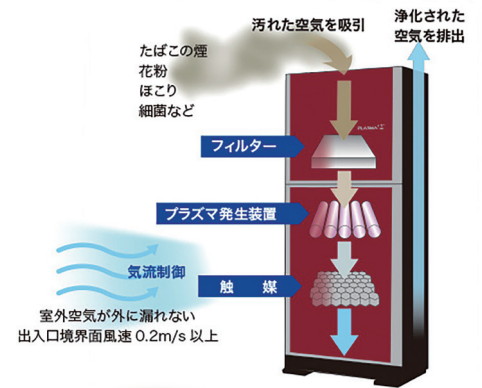
喫煙室用プラズマ脱臭機
