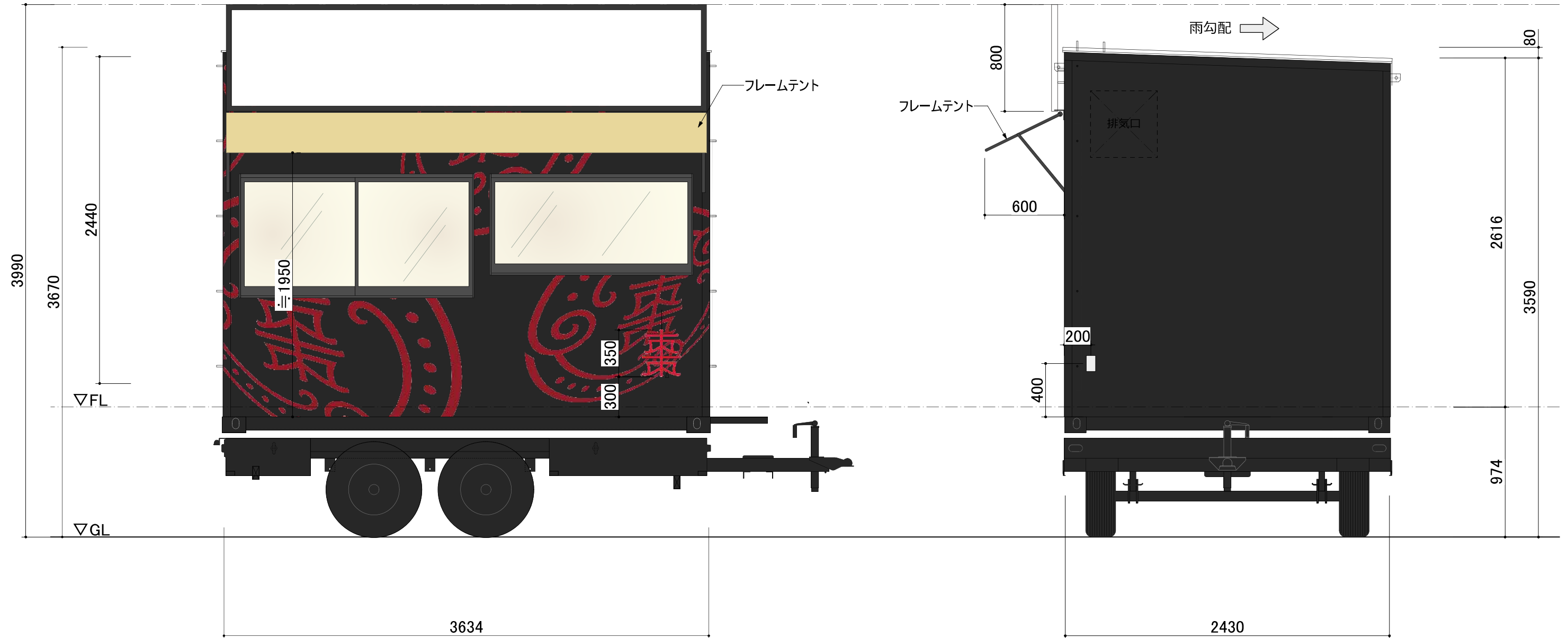
水上側 立面図
