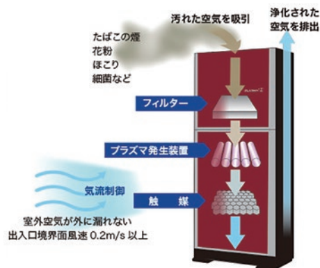
喫煙室用プラズマ脱臭機
