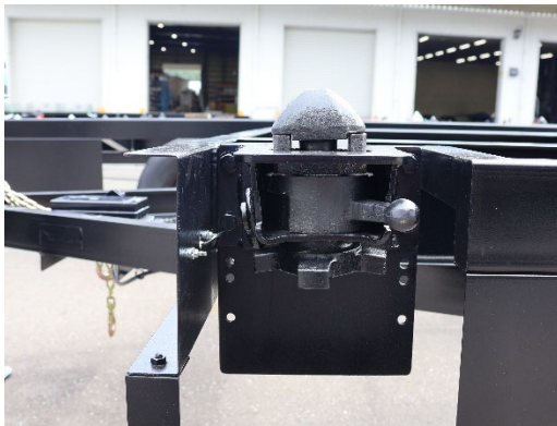
可変式コンテナロック
